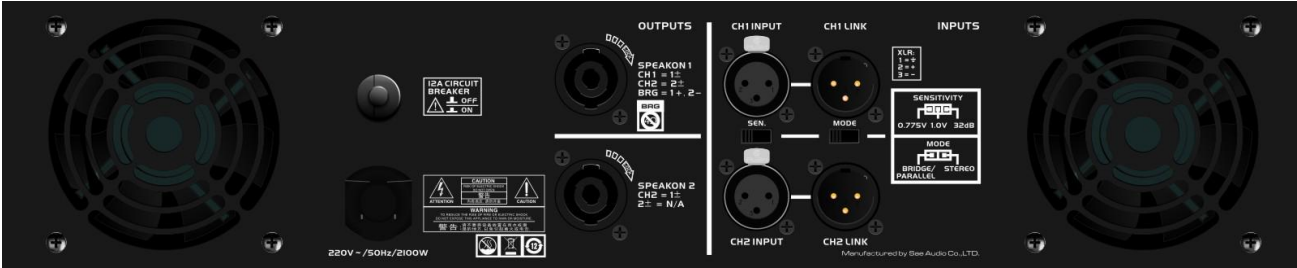
后面板
